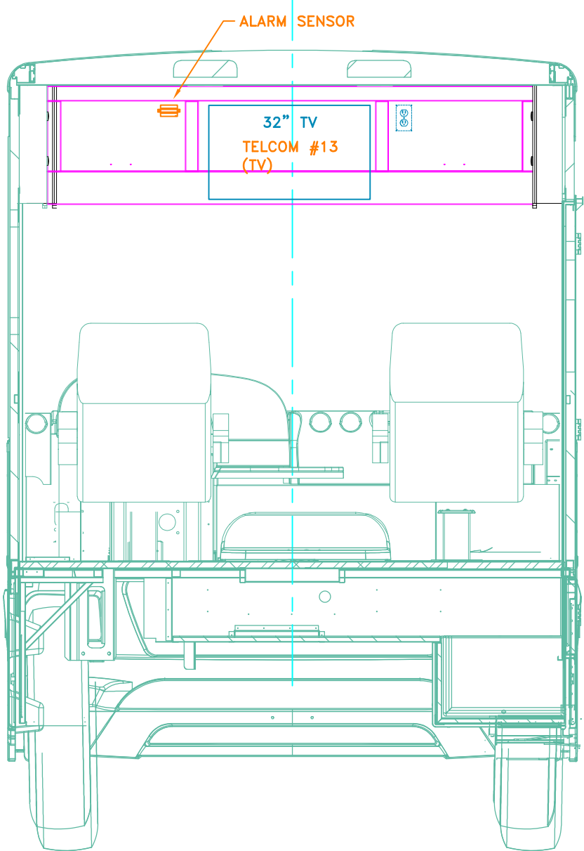
SECTION D-D
